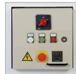
Ovládací panel s nastavitelným počítadlem klonků.
